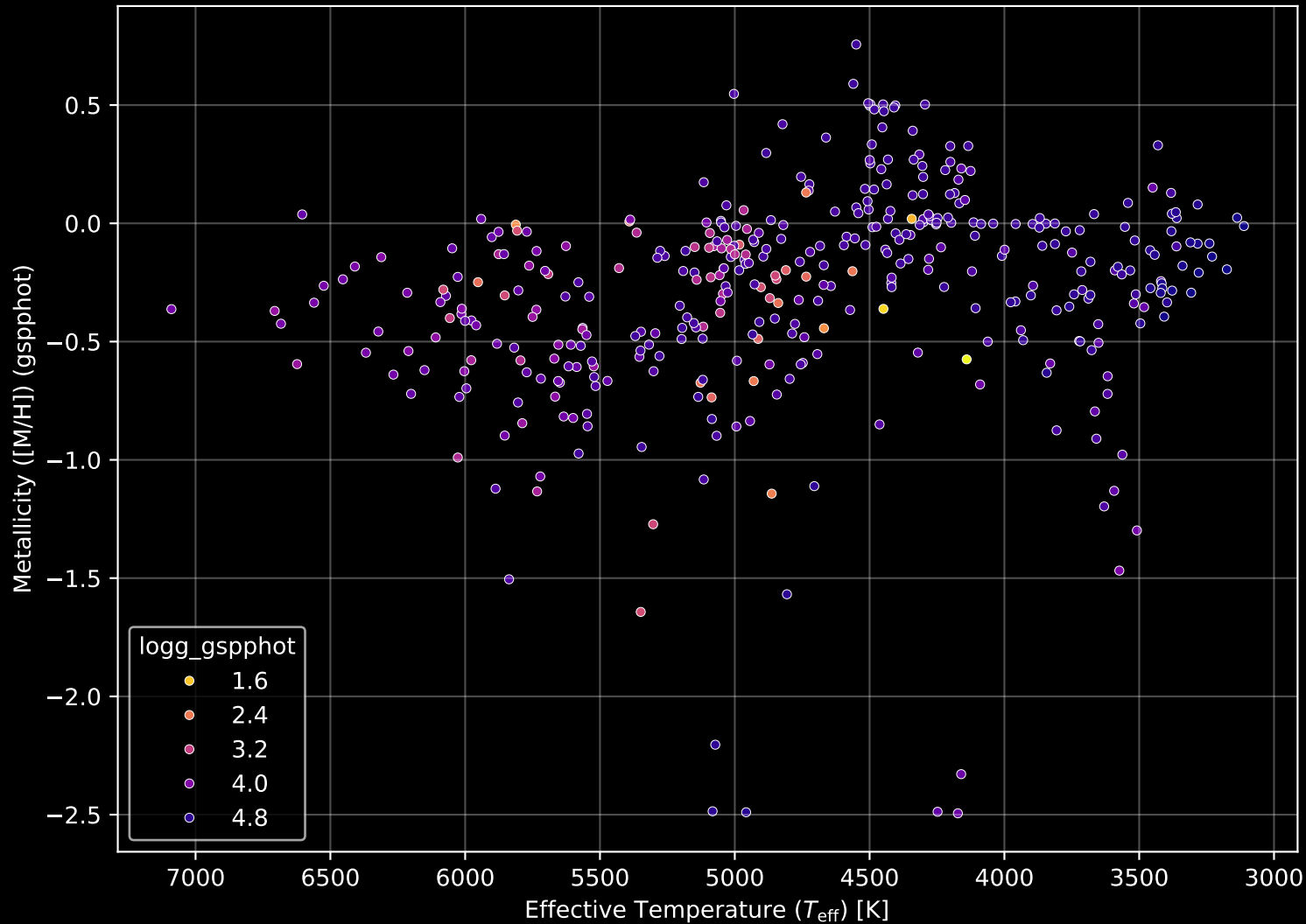
APOGEE DR17 Field: [180+75] Stellar Population Parameters (n= 398)
